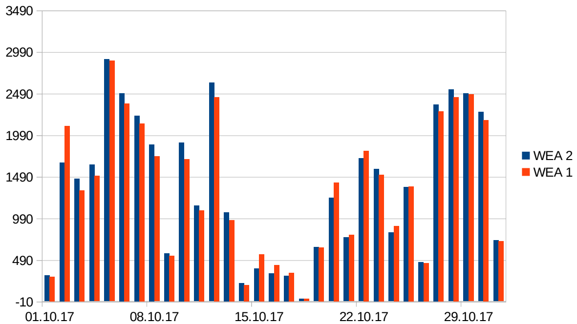
Durchschnittliche Anlagenleistung in kW
