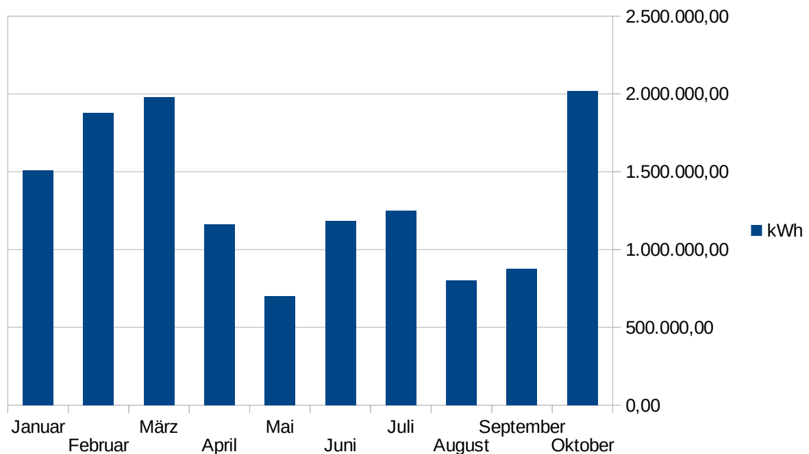
Energieertrag Jahresverlauf
