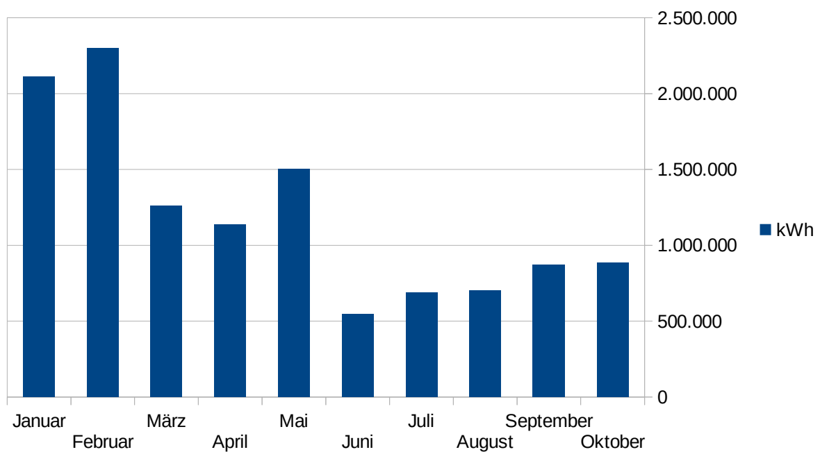
Energieertrag Jahresverlauf
