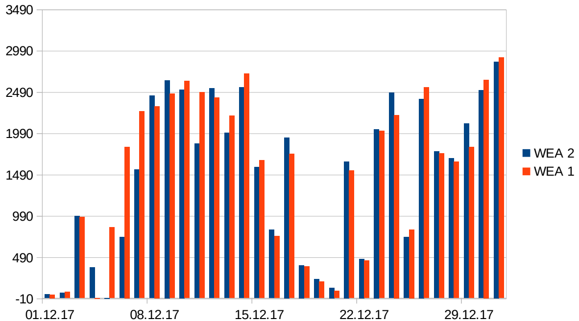
Energieertrag Jahresverlauf
